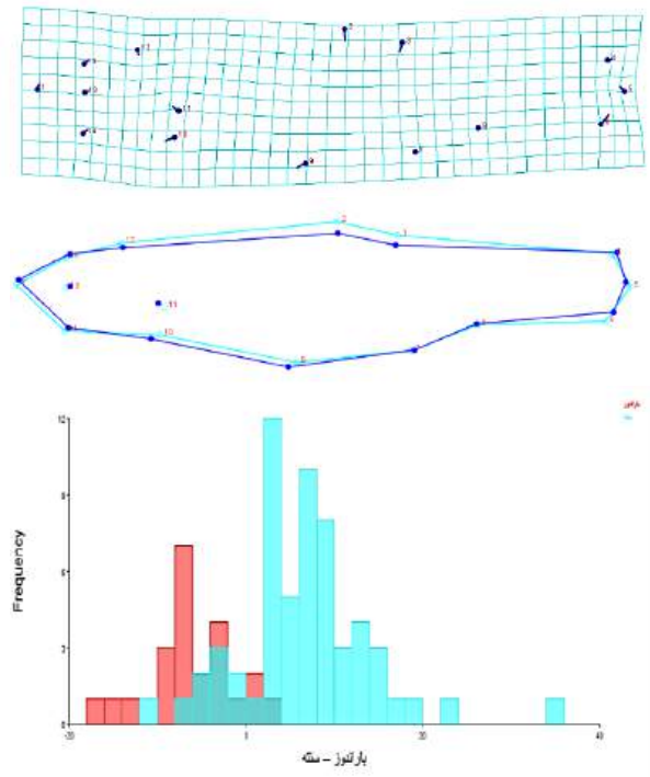
شکل ۱۳: مقایسه آنالیزهای چند متغیره (DFA) بین دو جمعیت رودخانه‌های باراندوز و سته
