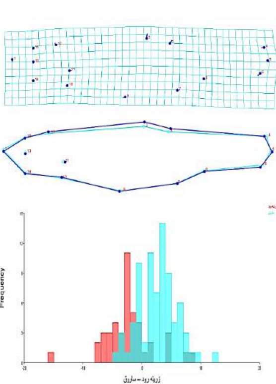
شکل ۱۹: مقایسه آنالیزهای چند متغیره (DFA) بین دو جمعیت رودخانه‌های زرینه‌رود و ساروق
