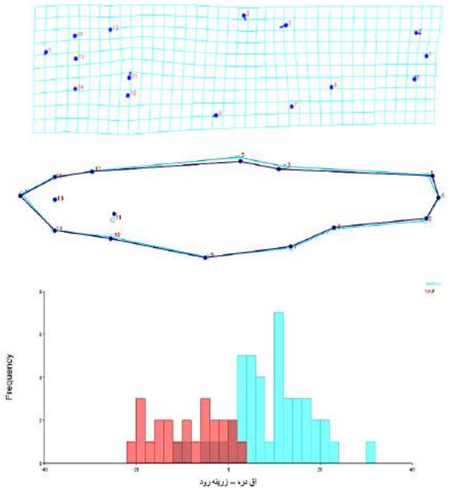
شکل ۶: مقایسه آنالیزهای چند متغیره (DFA) بین دو جمعیت رودخانه‌های آق دره و زرینه رود
