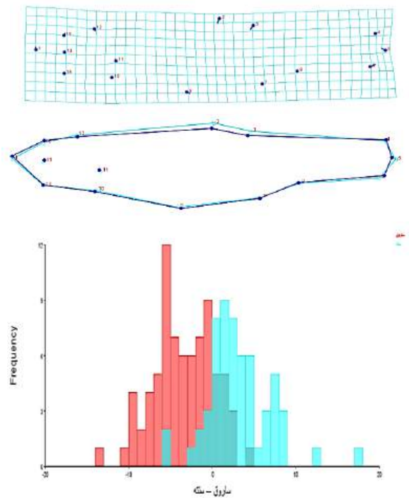
شکل ۲۲: مقایسه آنالیزهای چند متغیره (DFA) بین دو جمعیت رودخانه‌های ساروق و سنته
