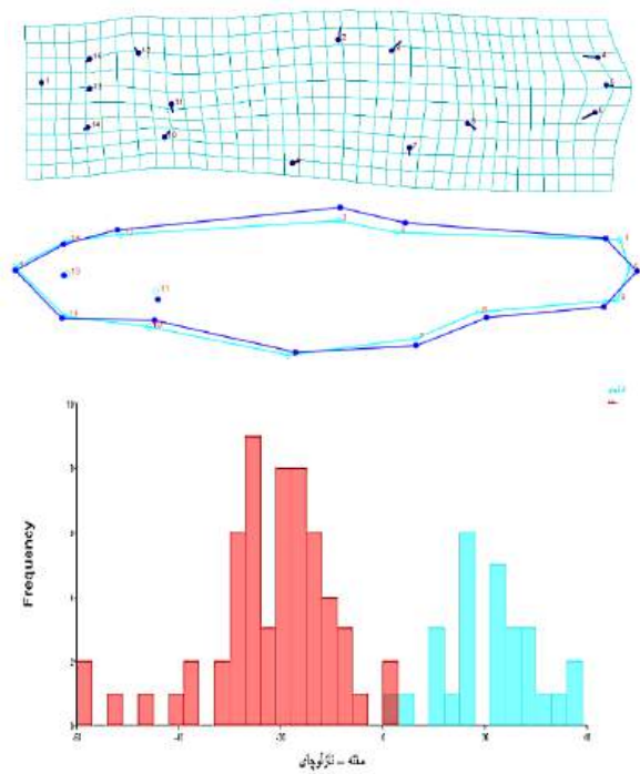
شکل ۲۴: مقایسه آنالیزهای چند متغیره (DFA) بین دو جمعیت رودخانه‌های سنته و نازلوچای
