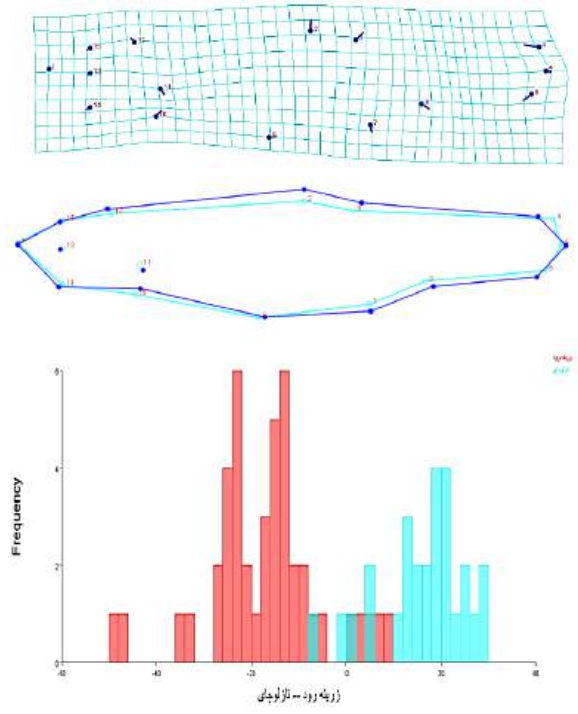
شکل ۲۱: مقایسه آنالیزهای چند متغیره (DFA) بین دو جمعیت رودخانه‌های زربنه رود و نازلوچای
